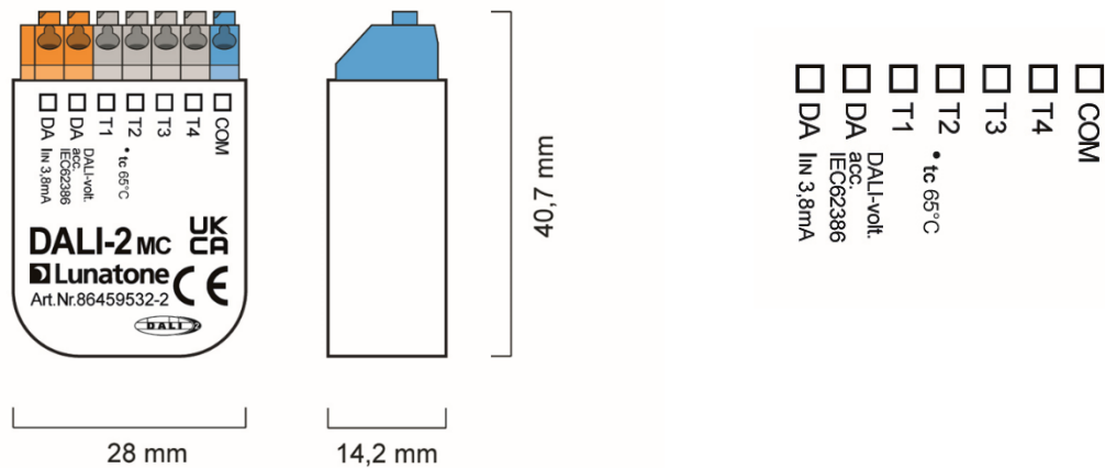
dimensions
